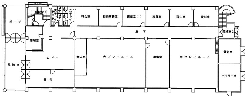
1階 平面図
