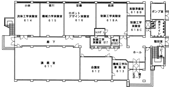
1階 平面図
